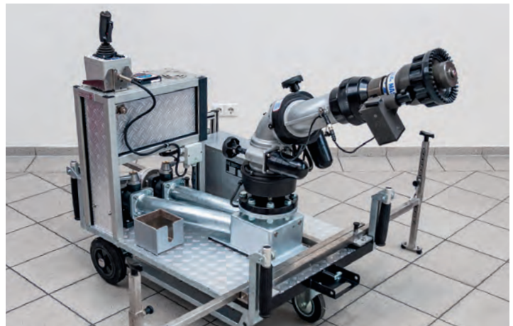
• Wasserwerfer Leader Vector, montiert auf fahrbarem TS-Modul.
